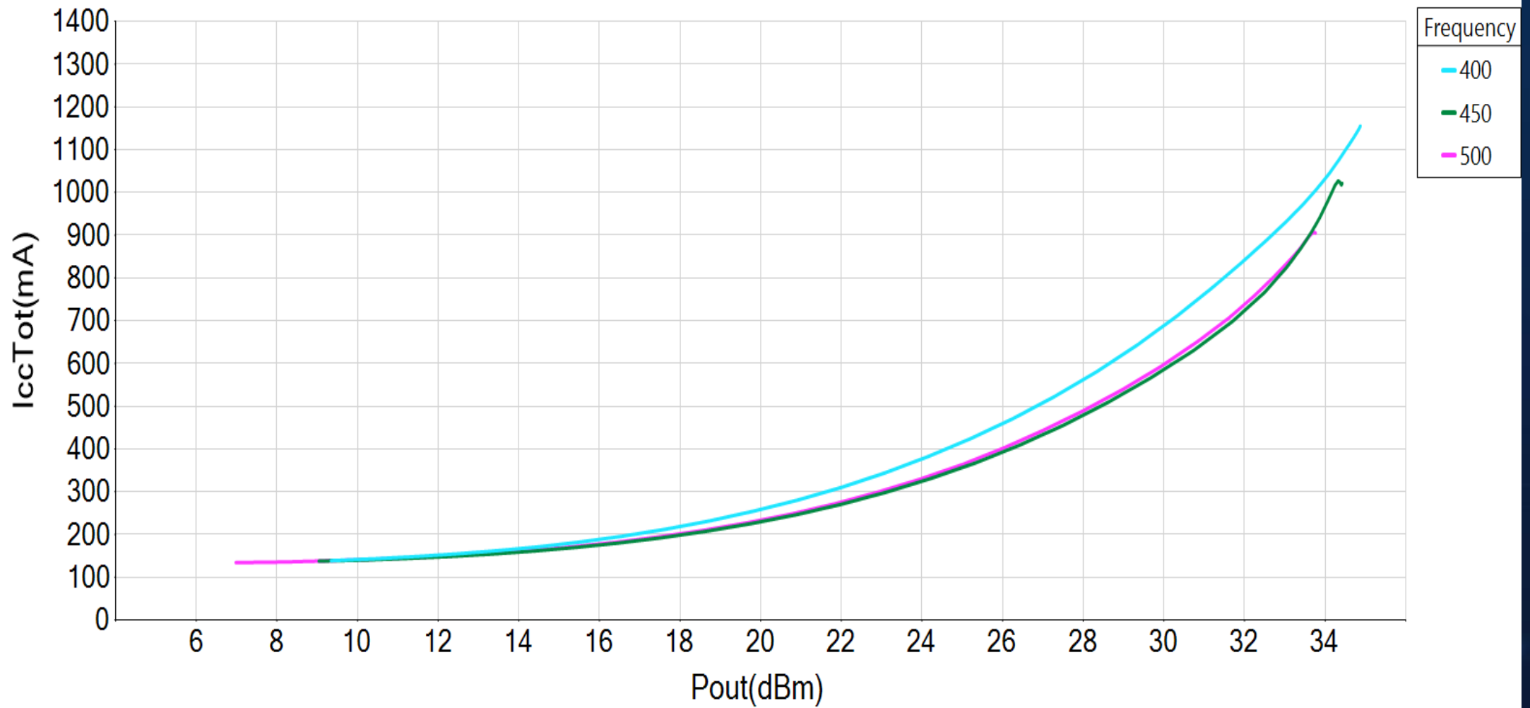
GRF5504 IccTot vs Pout
