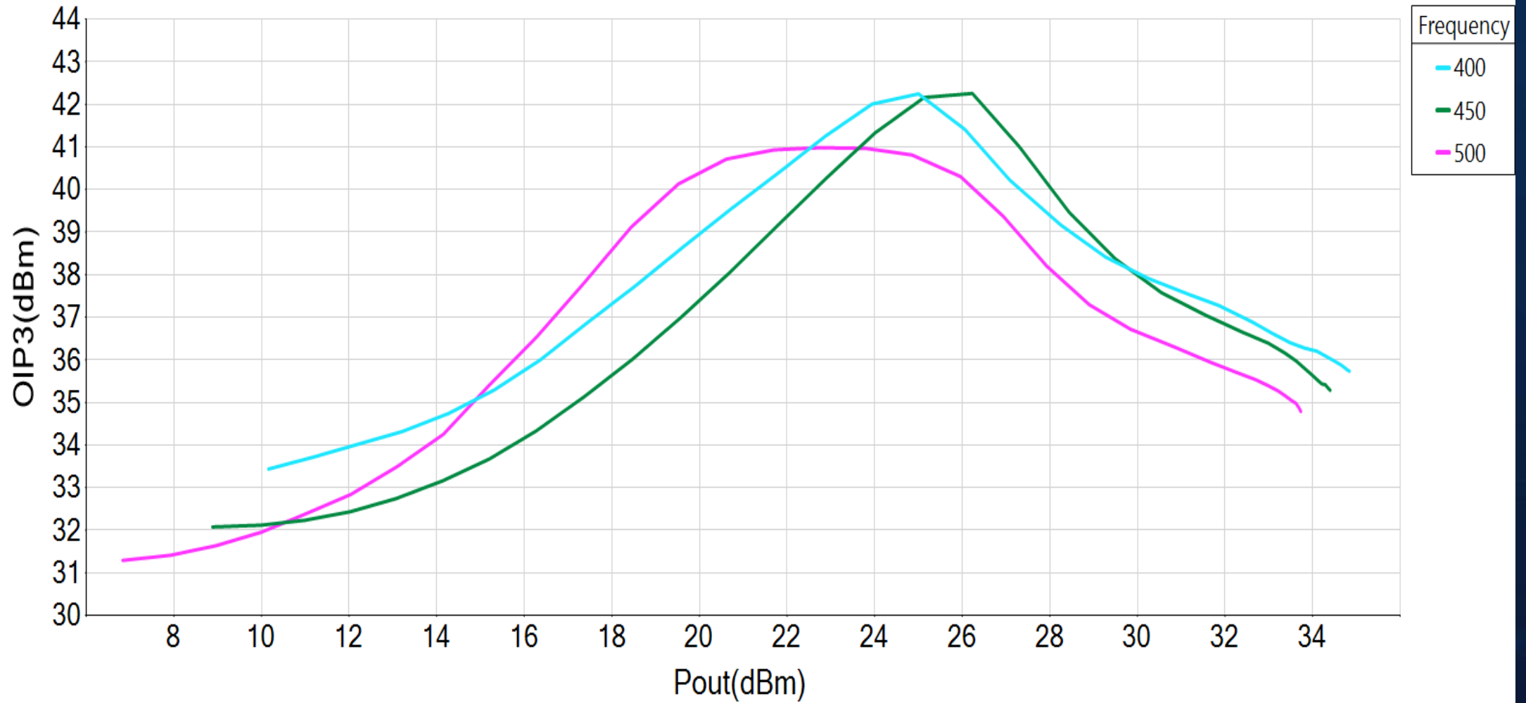
GRF5504 OIP3 vs Pout
